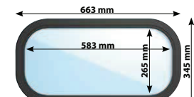
Abgerundete Ecken (r = 100 mm), hoher Isolierungswert
